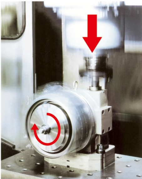
TILTING 230-150
